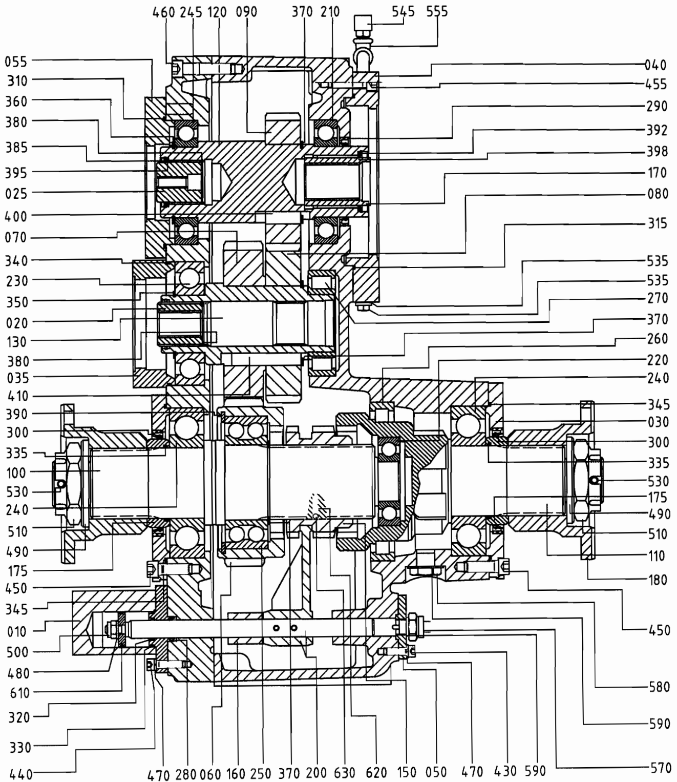
VIEW A-A
