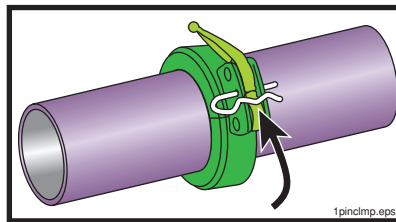
Figura 63 Póngale pasador a todas las abrazaderas
